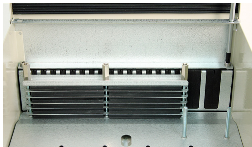
Hålbild i botten på Skarvskåp T4 96A-B Art nr. 11 470 220/225 Kabelgenomföring för upptill 6 kablar max 18 mm 96 st. mikrokabel/dukt 5-7 mm. Inkl. extra gummi- lamell låsning på insida.
