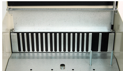
Hålbild i botten på Skarvskåp T4 60A-B Art nr. 11 470 223/224 Kabelgenomföring för upptill 6 kablar max 18 mm 60 st. mikrokabel/dukt 7 mm mekaniskt förankrade i slitsgavel.
