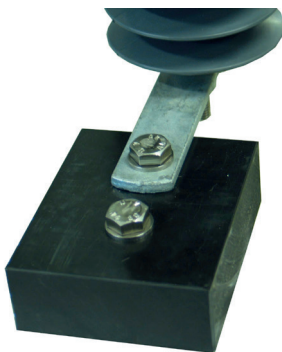
Isoleringskloss Skrues direkte i AL-travers
