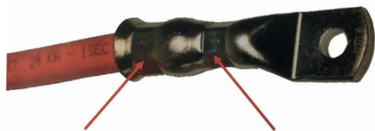
Press 2. Vanntetting over isolasjon
