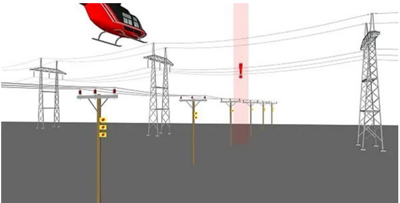
Merking av kryssende luftspenn: REN anbefaler skilt for markering av kryssende overliggende luftspenn. Illustrasjon hentet fra RENblad 8032 - Versjon: 1.10
