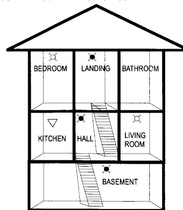
FIGUR 2 – TO/TREETASJES HUS
